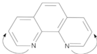
фенантролин
